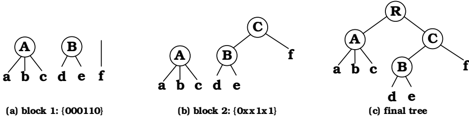
Fig. 4. Decoding AVT.
